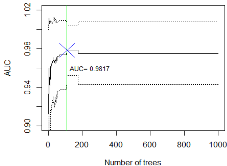
Fig. 3. Parameter tuning: Model 2
