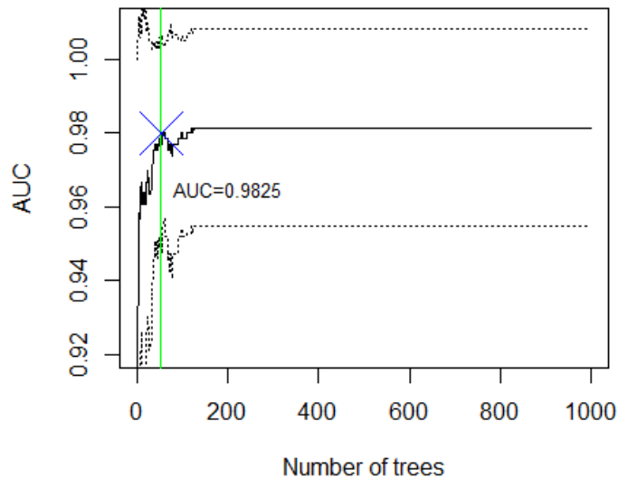
Fig. 4. Parameter tuning: Model 3 (final model)
