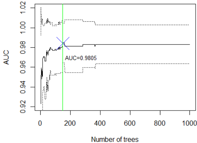
Fig. 2: Parameter tuning: Model 1
