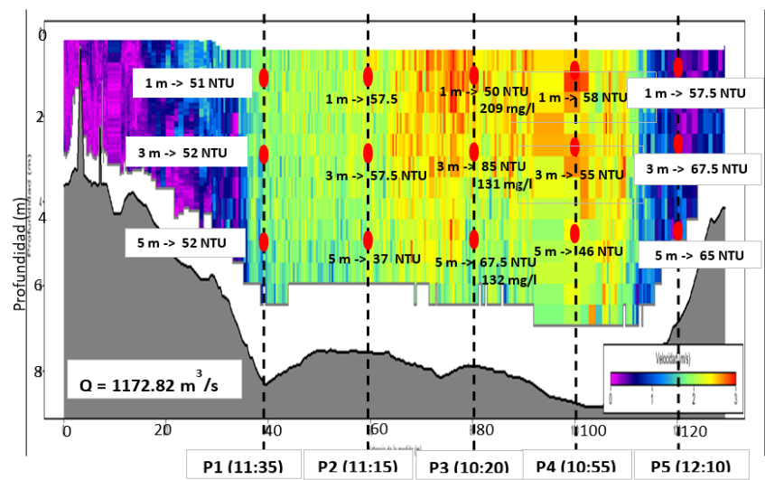
Figura 7 | S1, Puente de Ascó. Campo de velocidad, turbidez y concentración en los puntos de muestreo.
