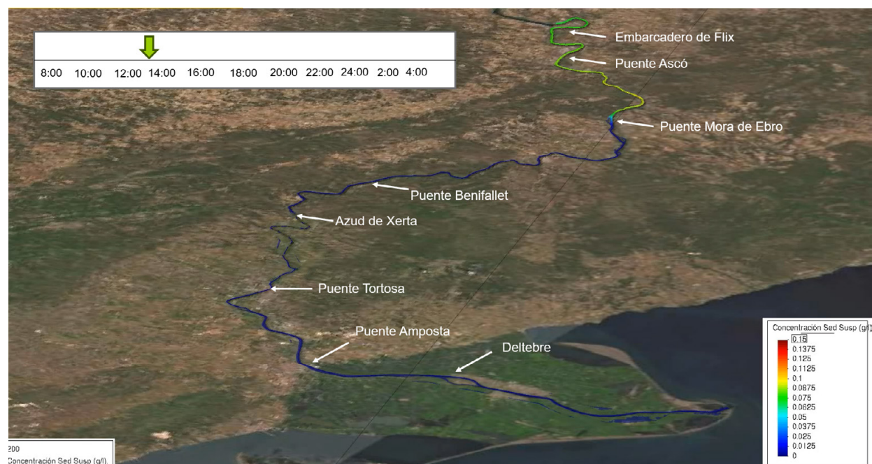
Figura 10 | Simulación numérica Iber. Campo de concentración de sedimentos en suspensión a las 13:40 horas.
