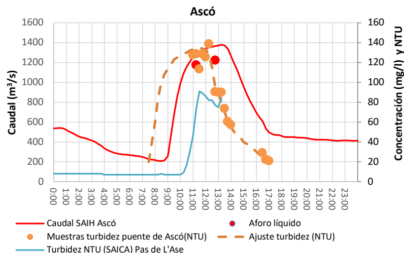
Figura 9 | S1, Hidrograma y registro de turbidez en Ascó.
