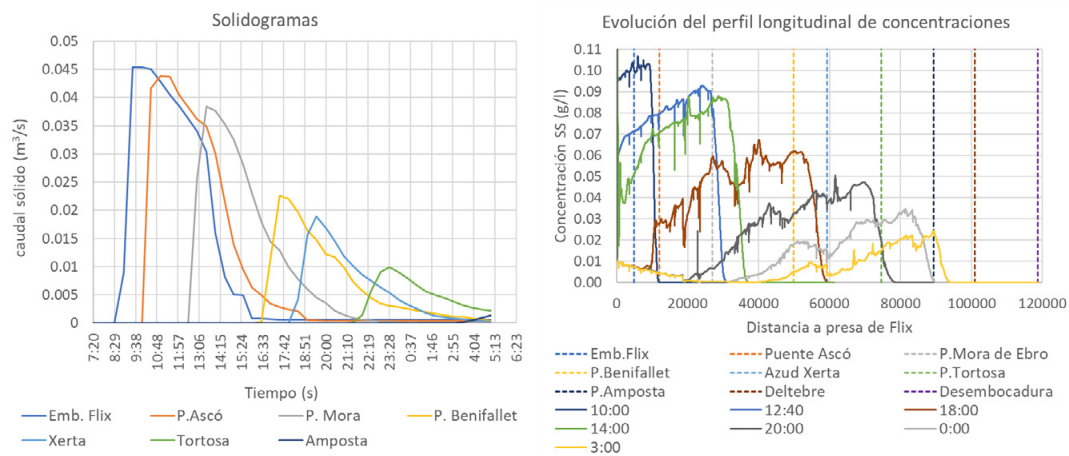
Figura 11 (continuación) | Principales resultados de la modelización del transporte de sedimentos realizada con el modelo Iber.
