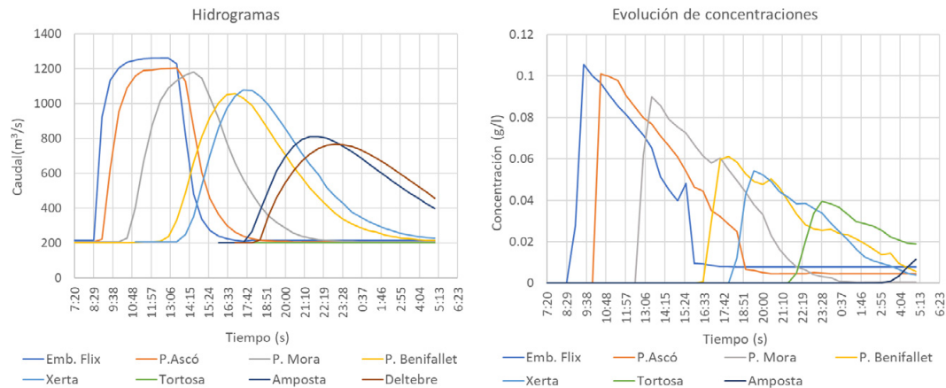
Figura 11 | Principales resultados de la modelización del transporte de sedimentos realizada con el modelo Iber.
