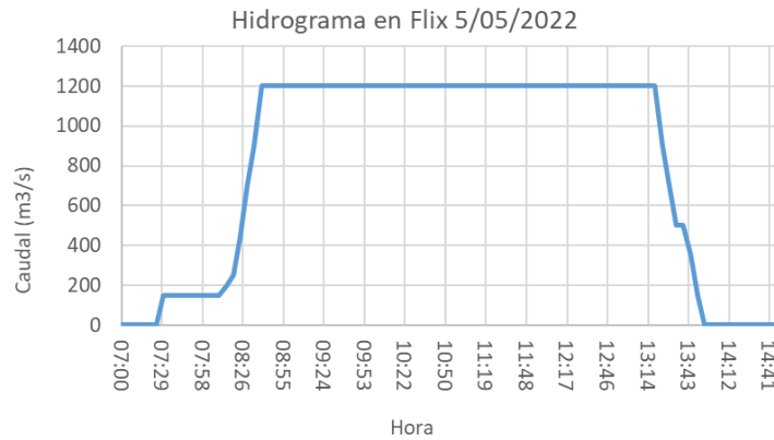
Figura 3 | Hidrograma programado de la avenida controlada desde Ribarroja.
