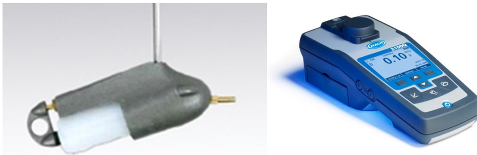
Figura 4 | Turbisonda modelo USB-48, Bureau Reclamation (izquierda). Turbidímetro (derecha).
