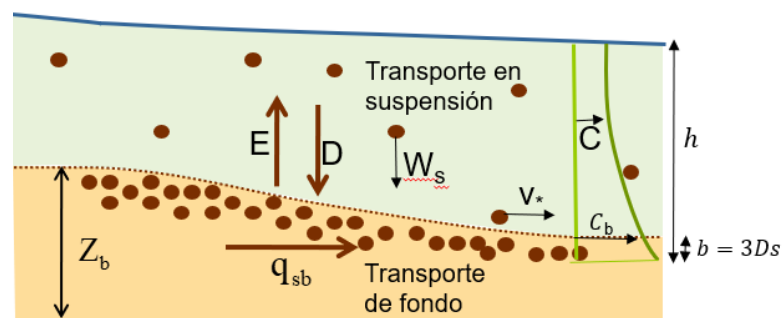
Figura 2 | Esquema de la ecuación de Exner para determinar la evolución del lecho.
