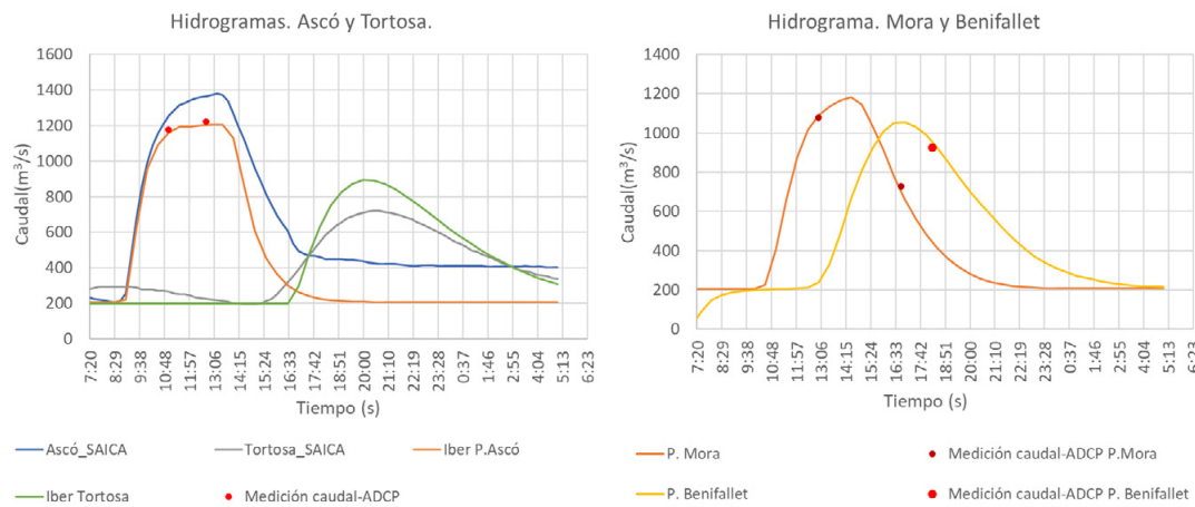
Figura 12 | Validación de caudales obtenidos con el modelo Iber.
