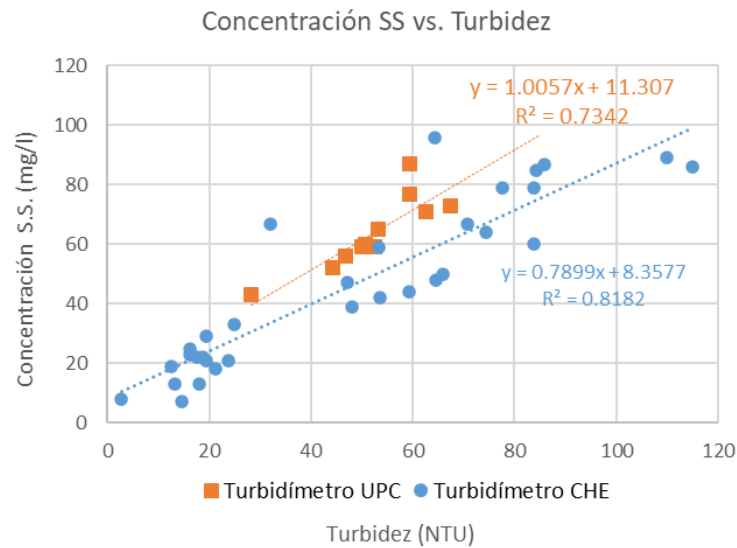
Figura 8 | Relación entre la turbidez y la concentración de sólidos en suspensión en los puntos de muestreo.
