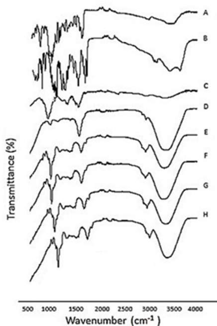
Fig. 2. FT-IR spectra of A) naringin; B) mangiferin; C) sodium hyaluronate; D) ultra-deformable-liposomes; E) glycosomes; F) et-glycosomes; G) glycerohyalurosomes; H) et-glycerohyalurosomes.
