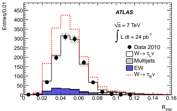
(c) EM radius
