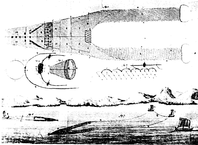
5. A finals del set-cents, l'únic gànguil en servei pescava en l'Albufera de València. La xarxa d'arrossegament, els components de la qual es detallen en la part superior de la imatge, era arrossegada per una o dues embarcacions segons les dimensions de l'art (Sáñez, I, 225)
