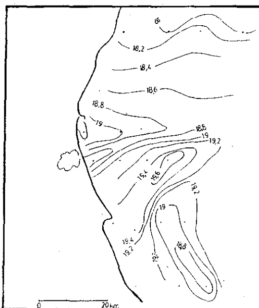
Fig. 14.—Temperatura superficial del mar durante la campaña Plataforma V (31 mayo-4 junio 1980). (Elaborado a partir de los datos del Informe Científico.)
