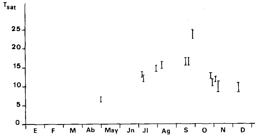
Fig. 9 Evolución anual de la temperatura registrada por el satélite (máxima-minima) (°C) en el Golfo de Valencia.
